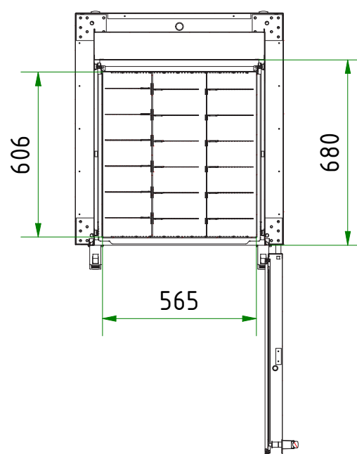
A-A ( 1 : 20 )
