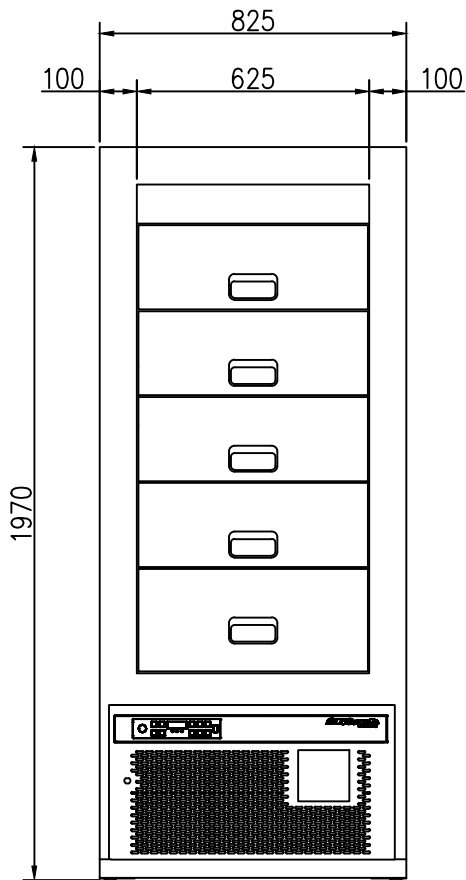
Ansicht ohne Türe gezeichnet
