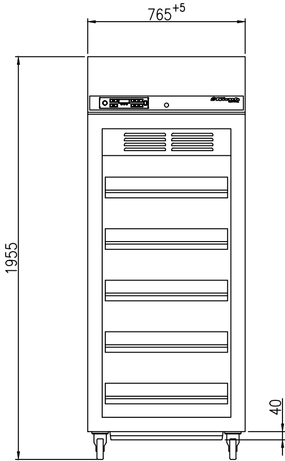
Ansicht ohne Türe gezeichnet
